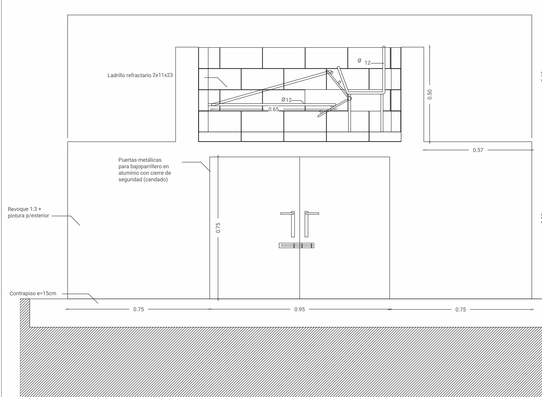
1 Parrillero A107 1:10
